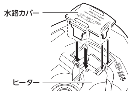
水路カバー
